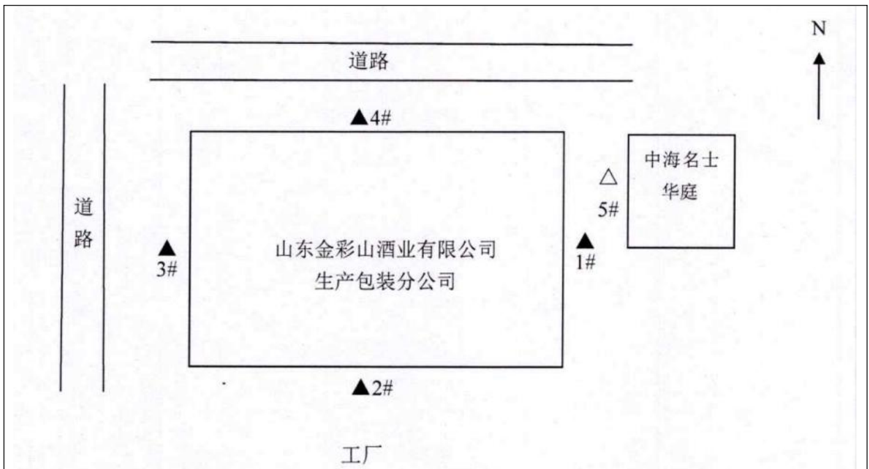
图 3-2 厂界及敏感点噪声监测点位示意图
