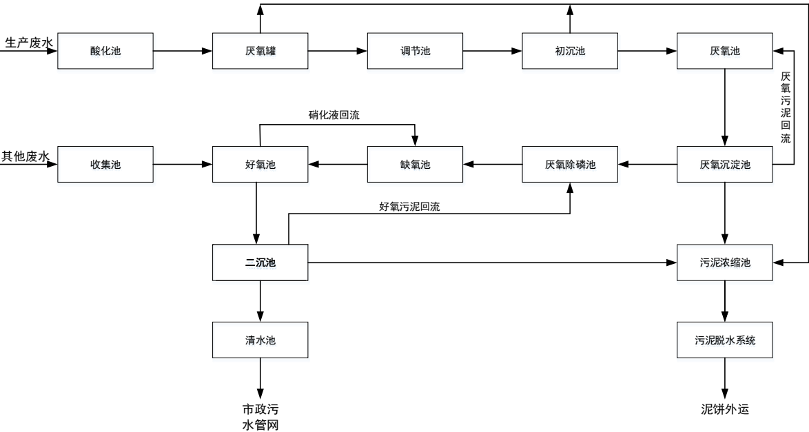
图 3-1 现有工程污水处理工程工艺流程图
